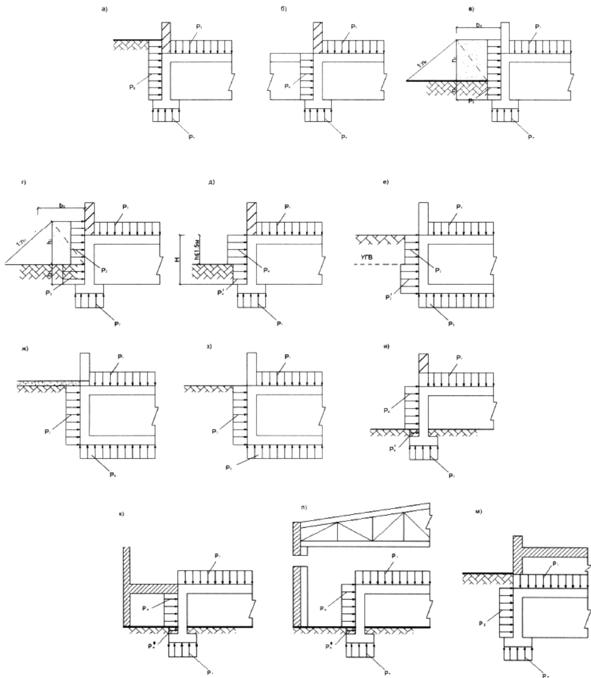
Рисунок 7.1 - Схемы приложения динамических нагрузок на конструкции убежищ
